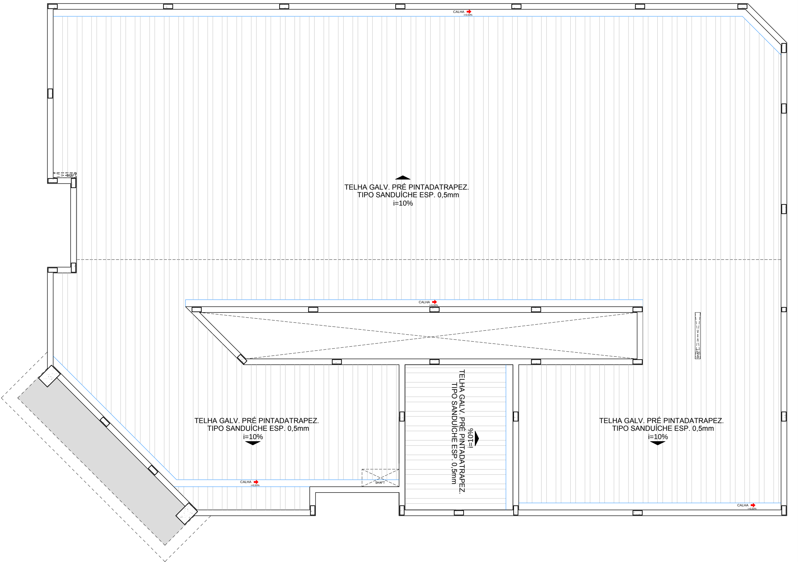
PLANTA COBERTURA ESCALA 1:100
