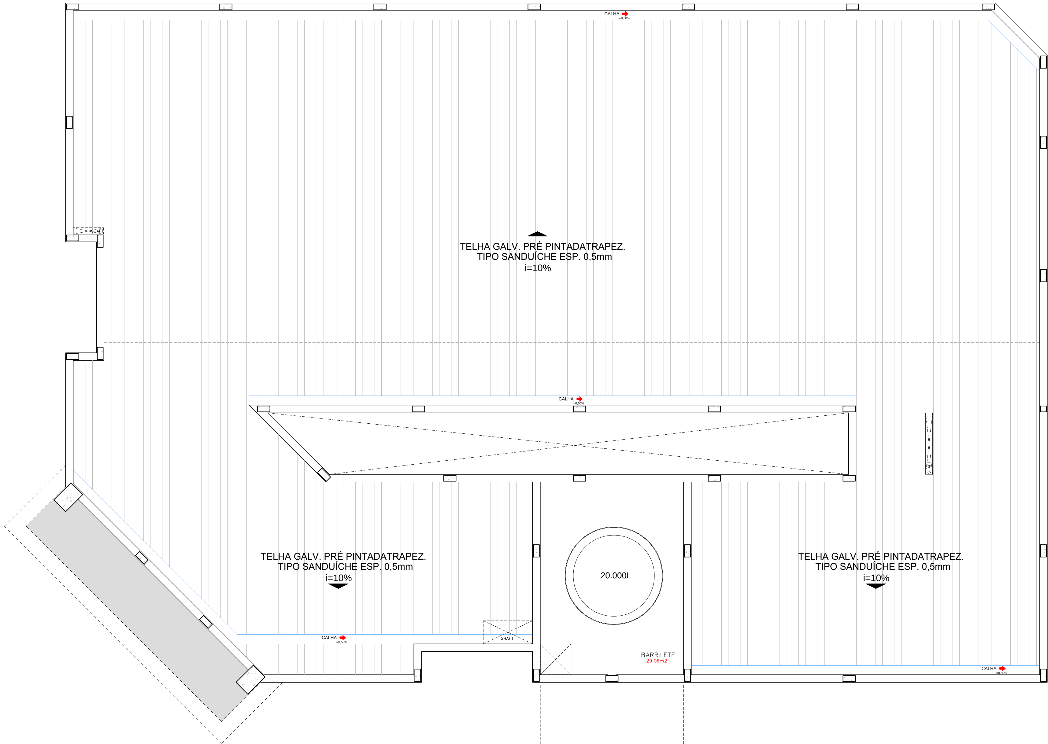
DETALHE BARRILETE ESCALA 1:75
